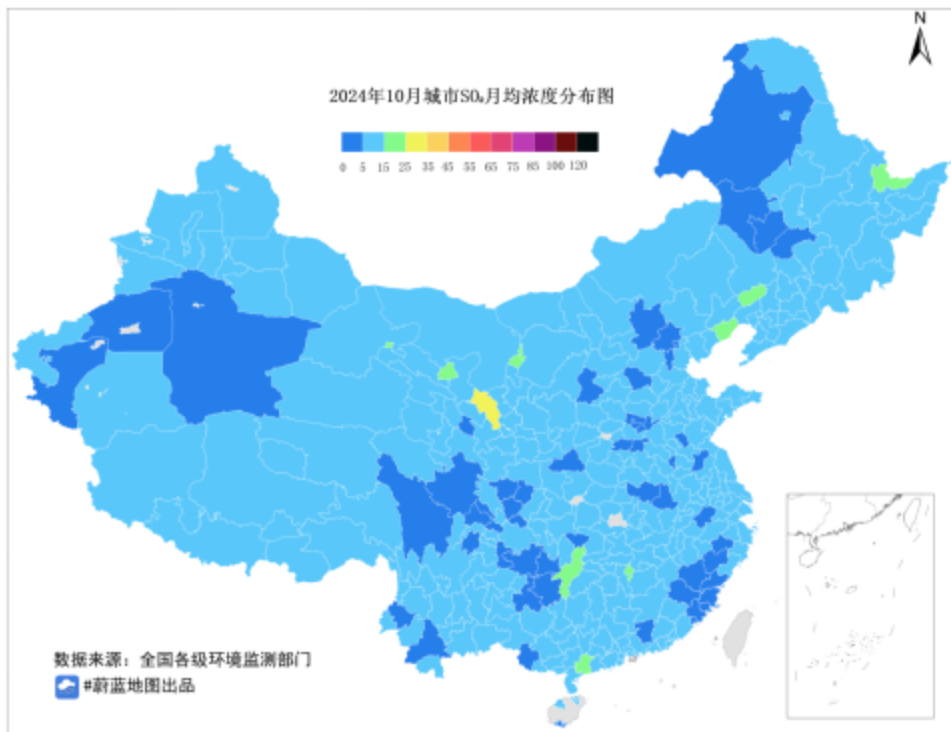
图 4 2024 年 10 月城市 SO_2 月均浓度分布图
