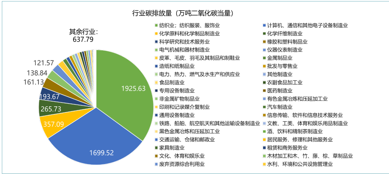
图 4-5：本评价期通过蔚蓝地图披露碳数据的行业排放量分布（万吨二氧化碳当量）
