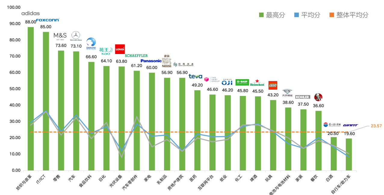
图 3-2：2024 CATI 行业得分对比
