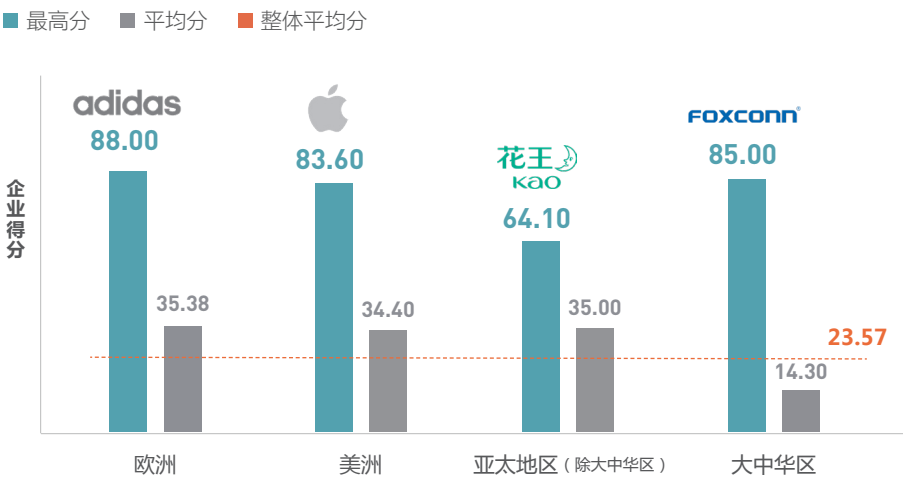
图 3-2：2024 CATI 区域得分对比
