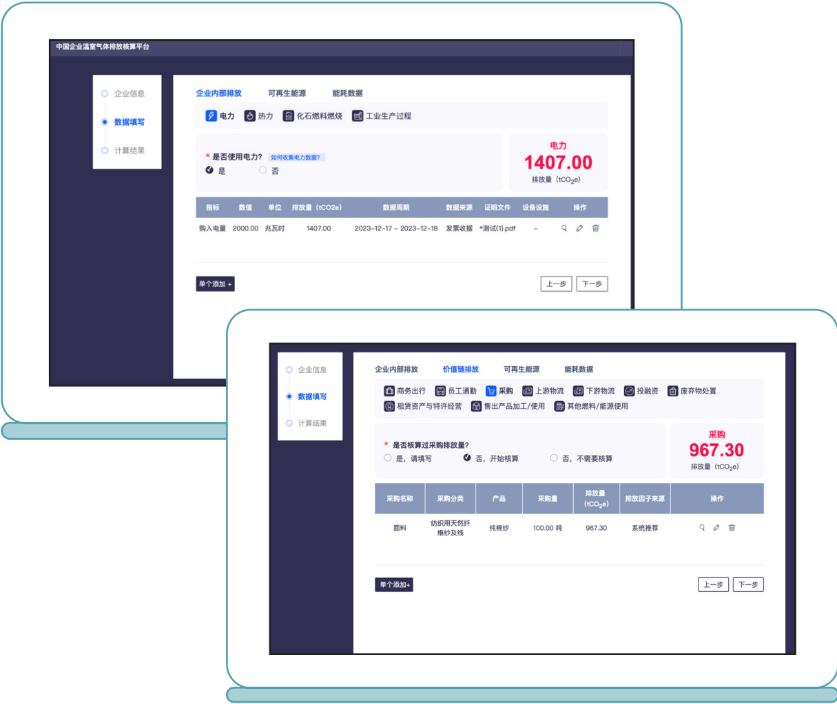
图 4-24：中国企业温室气体排放核算平台 - 范围 3
