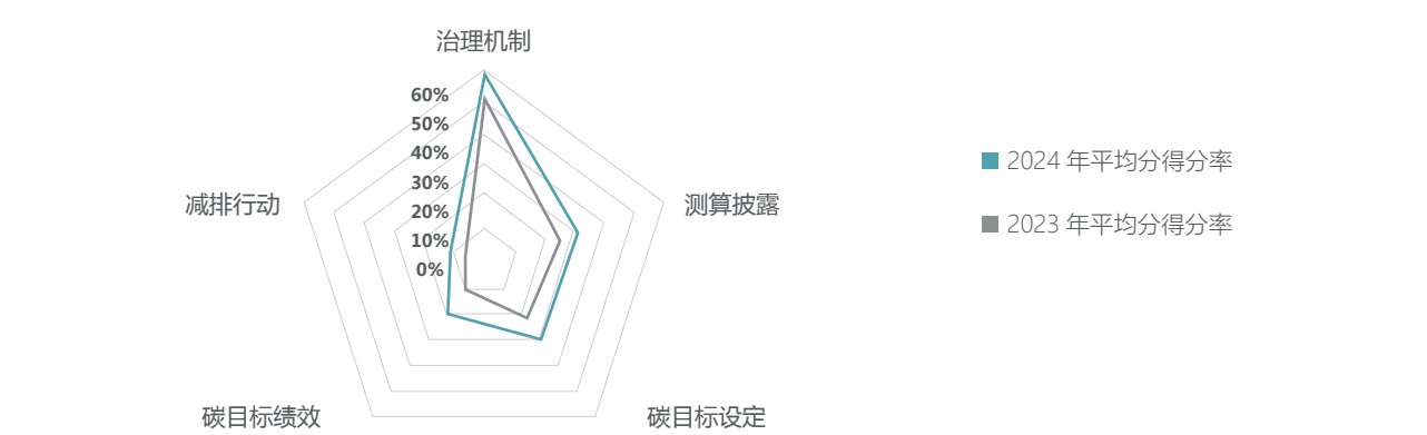
图 3-3：2023 与 2024 CATI 各维度平均得分率对比 9
