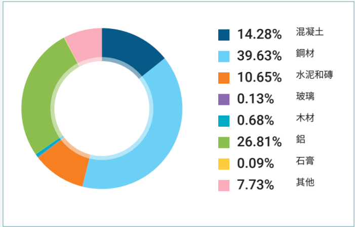
图 4-19：恒隆地产 2023 年不同建筑物料隐含碳排放占比
