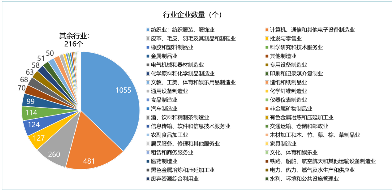
图 4-6：本评价期通过蔚蓝地图披露碳数据的供应商的行业分布（个）
