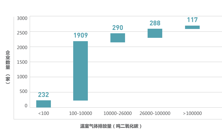
图 4-3：本评价期通过蔚蓝地图披露的碳排放数量级分布
