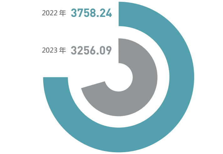
图 4-8：纺织、皮革和 IT/ICT 相关行业供应商 2023-2024 年排放量对比
