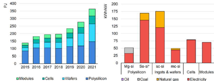
图 4-7：全球光伏产业能耗变化趋势及能源类型
