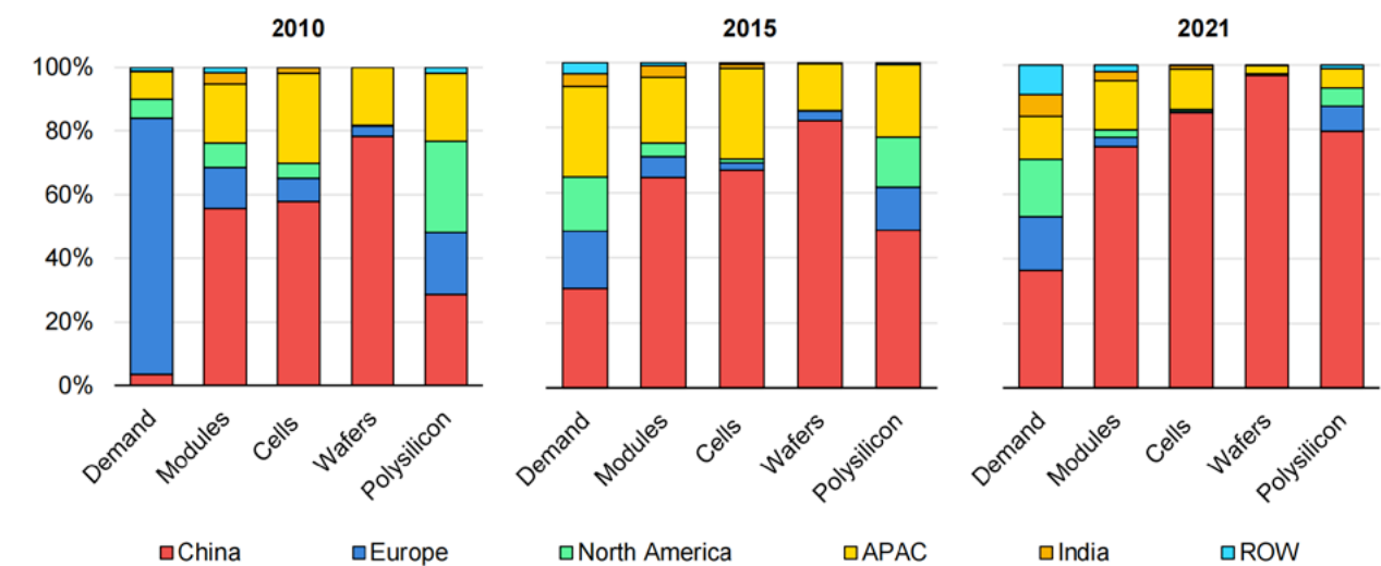
图 1-1：2010-2021 年按国家和地区分的太阳能光伏发电制造能力 17
