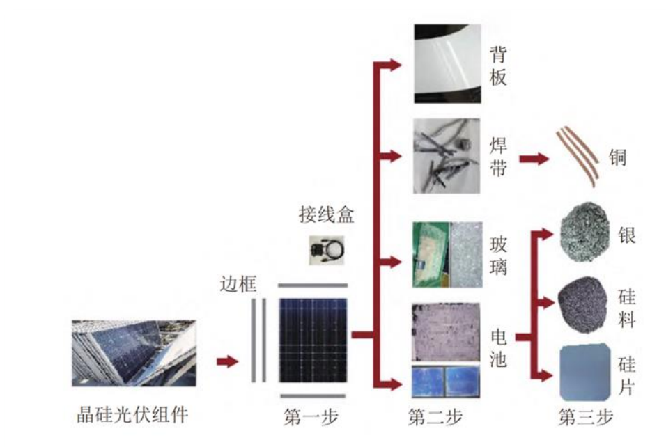
图 4-6 晶体硅光伏组件回收的一般流程 75
