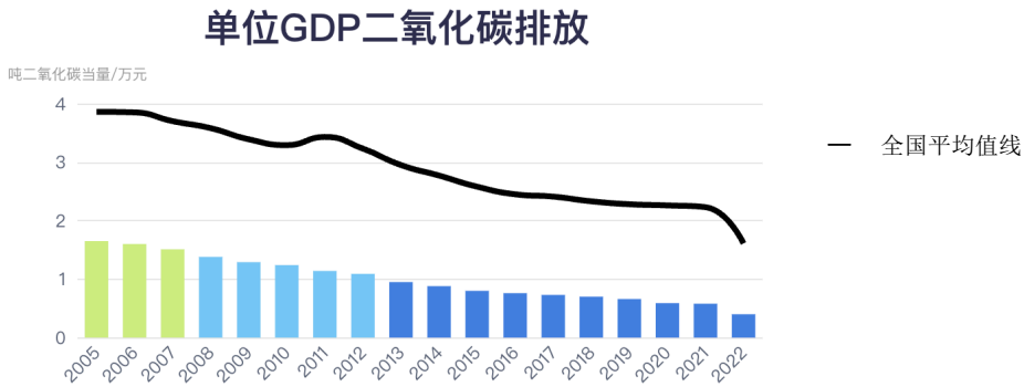
图 30 北京历年单位 GDP 碳排放强度
