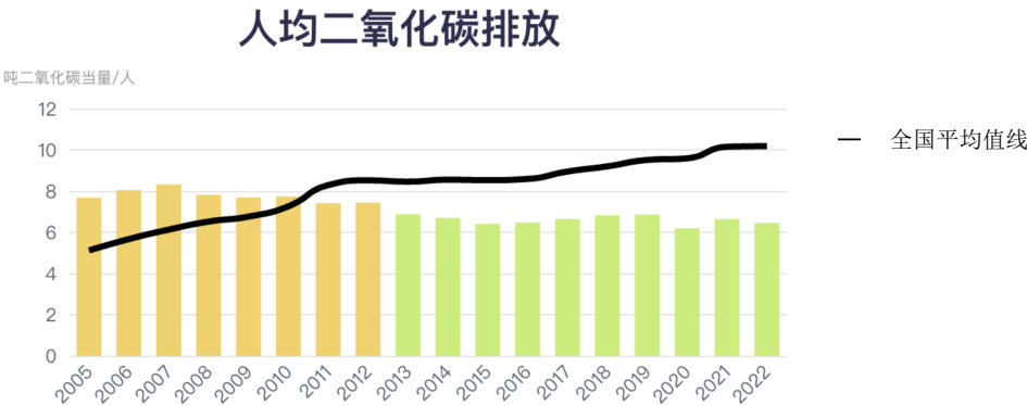
图 29 北京历年人均二氧化碳排放量
