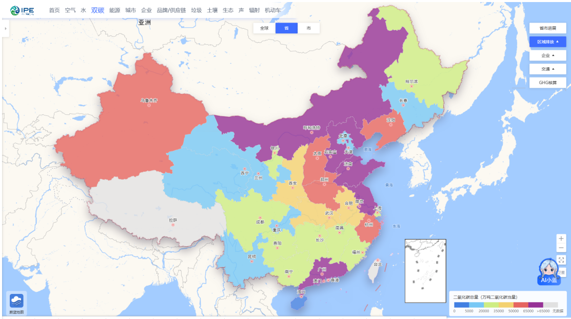
图 1 蔚蓝双碳地图（来源：IPE 网站）
