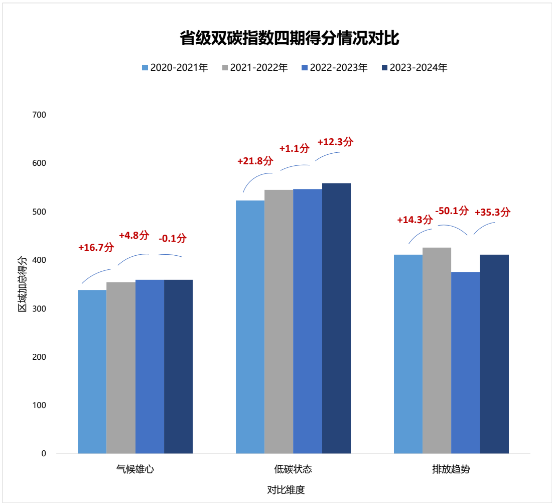
图 4 省级双碳指数四期得分情况对比图
