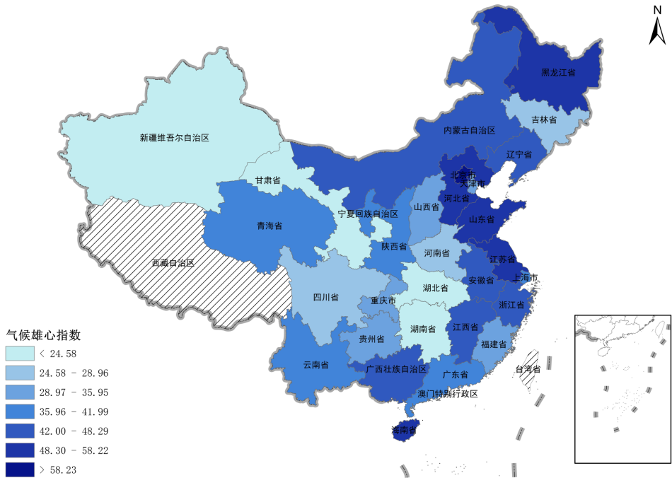
图 10 2022-2023 年度“气候雄心”分指数评价结果
