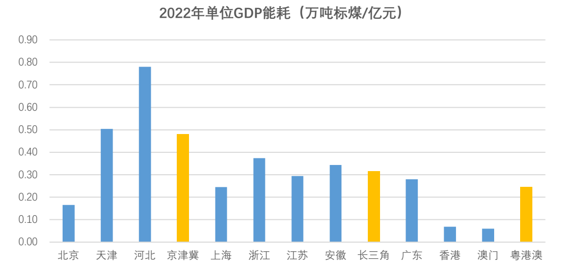
图 24 京津冀、长三角、粤港澳地区 2022 年单位 GDP 能耗情况
