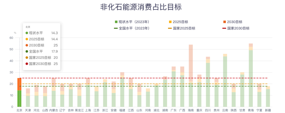
图 31 北京非化石能源消费占比现状水平
