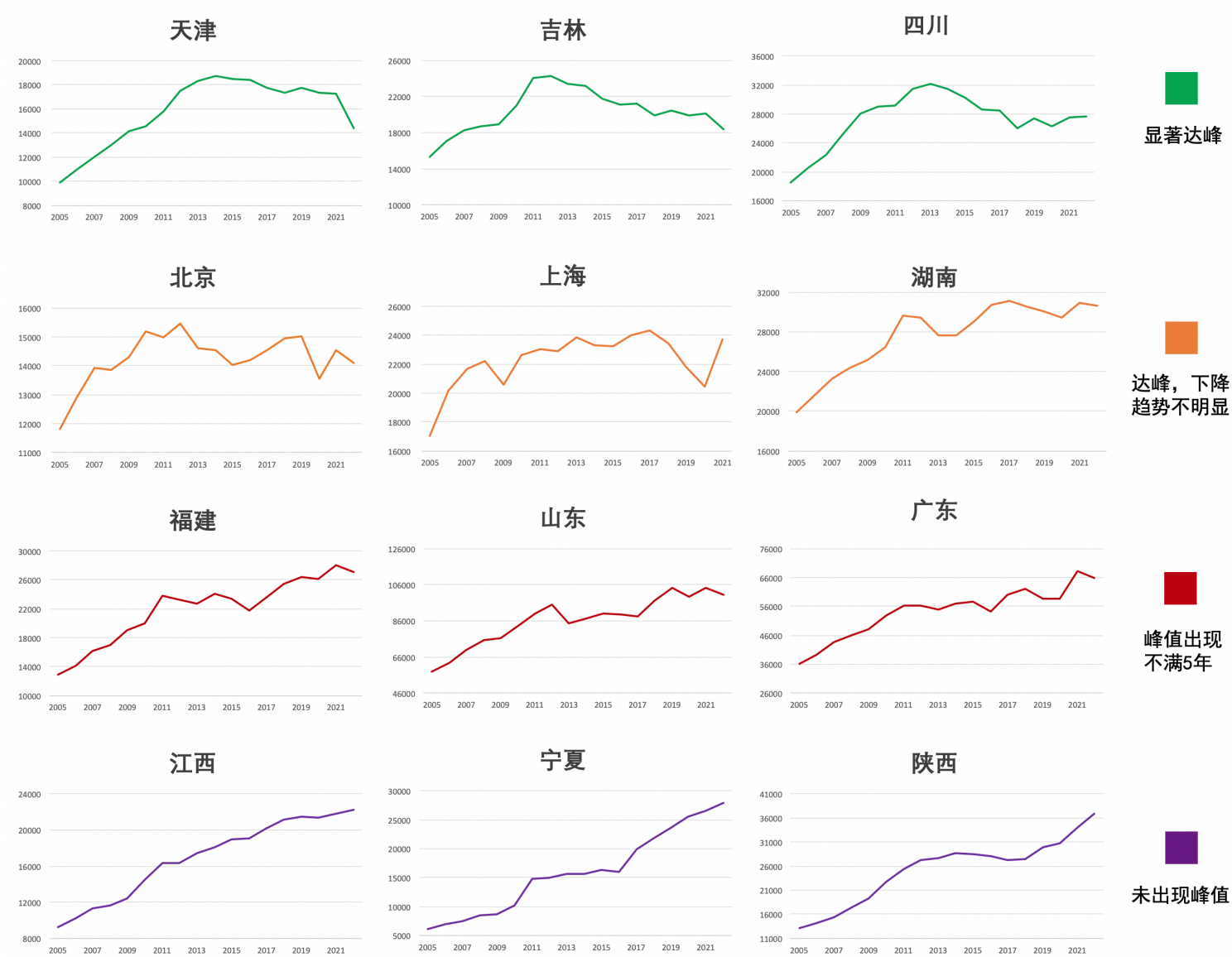
图 16 典型省级行政区碳排放趋势图
